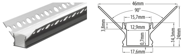
APG334 – прав профил
